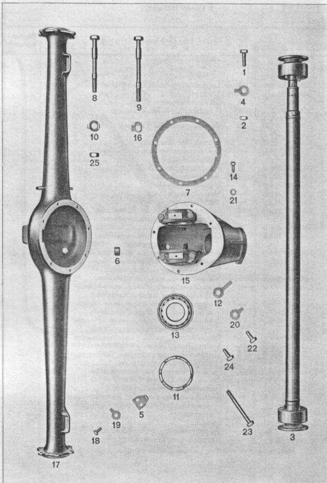
Tafel 29 Zwischenwelle, Hinterachsbrücke, Hinterachsgehäuse
