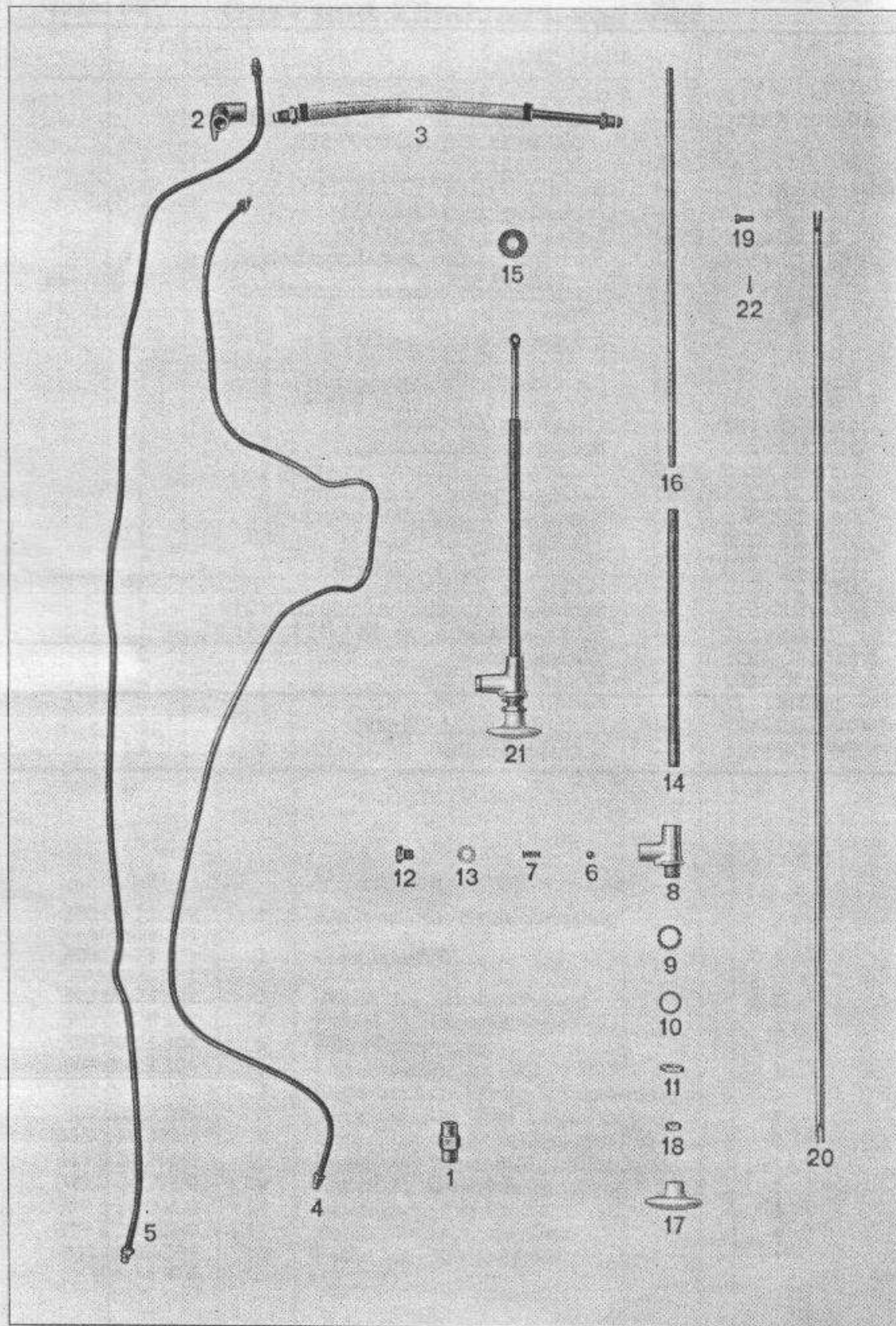
Tafel 37 Kraftstoffleitung, Handbetätigung der Kühlerjalousie
