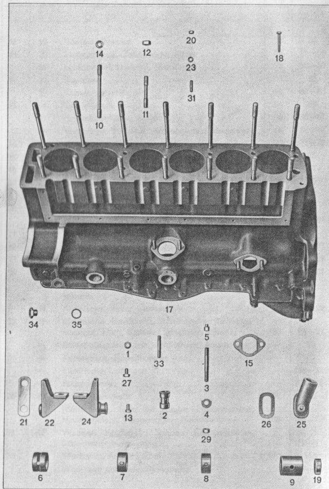
Kurbelgehäuse-Oberteil
